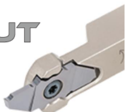
端面溝入れ
