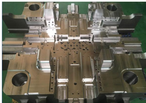
ダイカスト金型 (エンジン)
