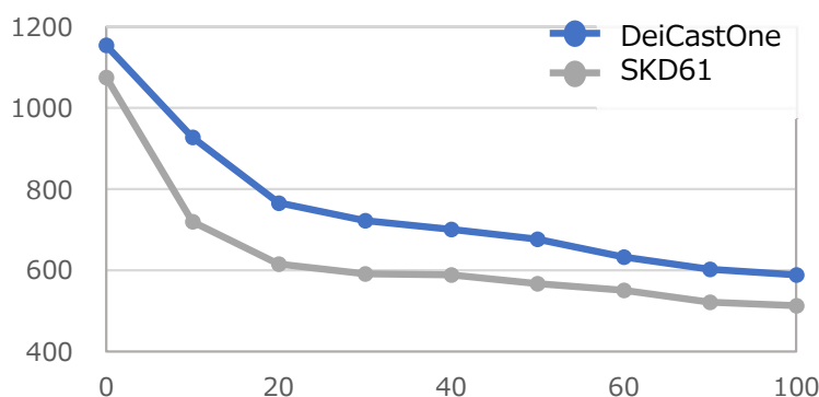
BGH DeiCast One材 硬さ分布
