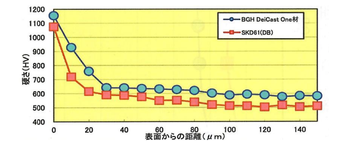
BGH Die-Cast One 処理後の硬さ分布
