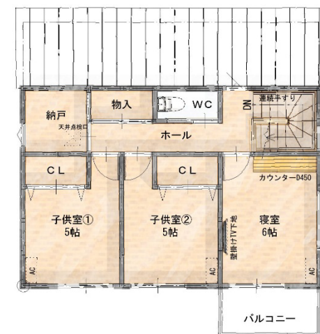
2F 平面図
