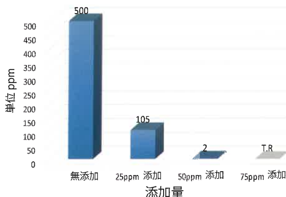
スーパーシュールス添加後の 残留硫化水素濃度
